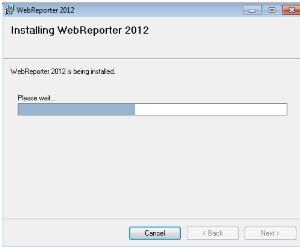
圖 8 – 安裝進度
