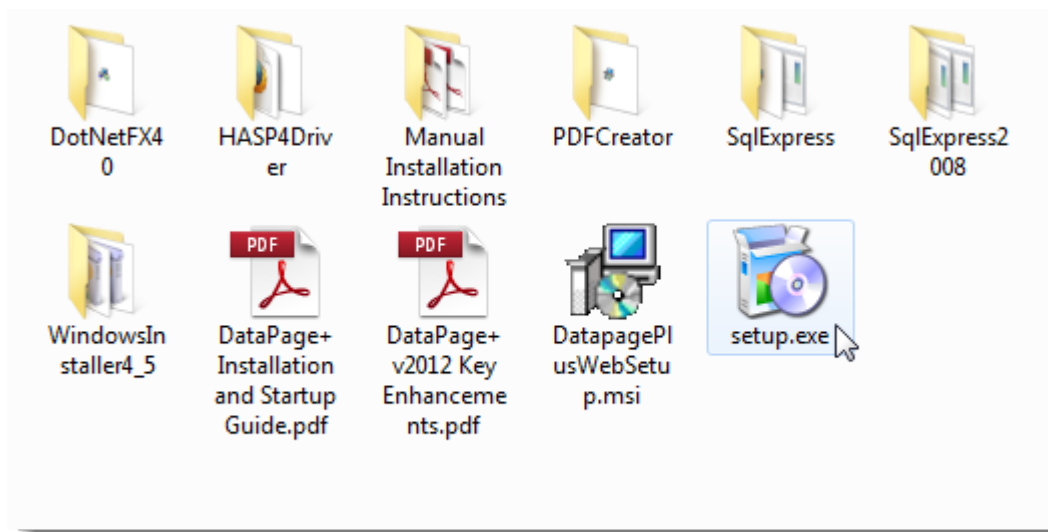
圖 2 – Setup.exe 檔案
